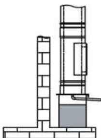
Stavitelný podstavec výškově stavitelný (založený na zemi)
