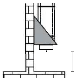
Založení na konzoli s čištěním spodem
